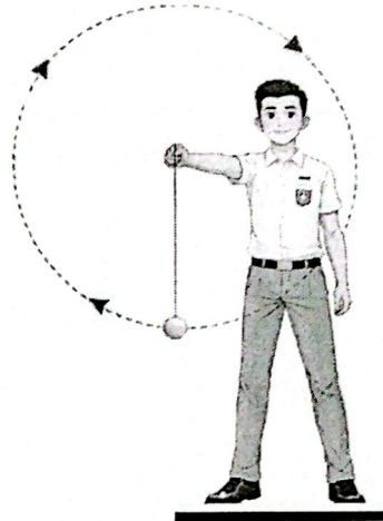
Gambar 1. Seorang Anak Memutar Bandul Secara Vertikal
